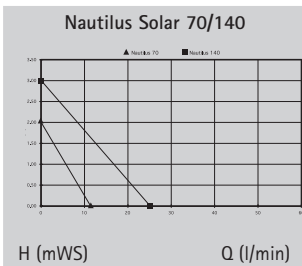
Pumpenkennlinie
