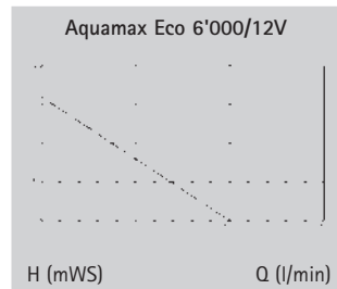
Pumpenkennlinie
